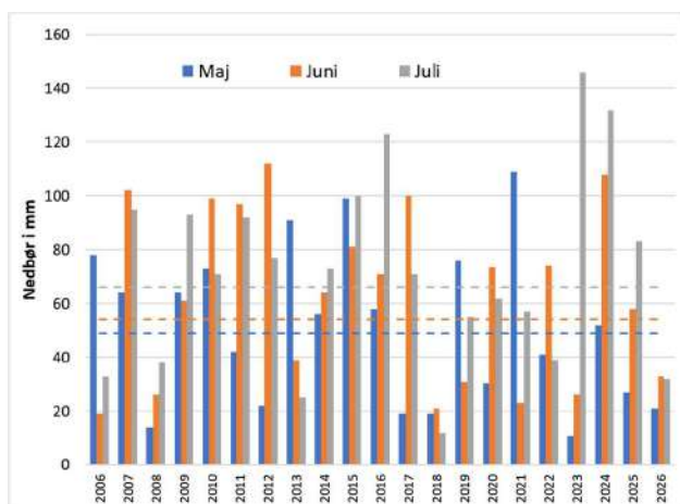
Figur 2a: Nedbør for månederne maj-juli 2006-2026 med normalerne indsat.
