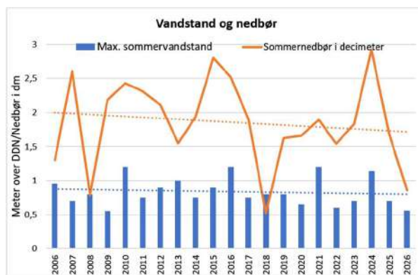
Figur 4b. Maksimal sommervandstand (maj-juli) over DNN målt i Århus Å opstrøms Brabrand Sø samt sommernedbør (maj-juli) målt i decimeter i perioden 2006-2026. Trendlinjer indsat.
