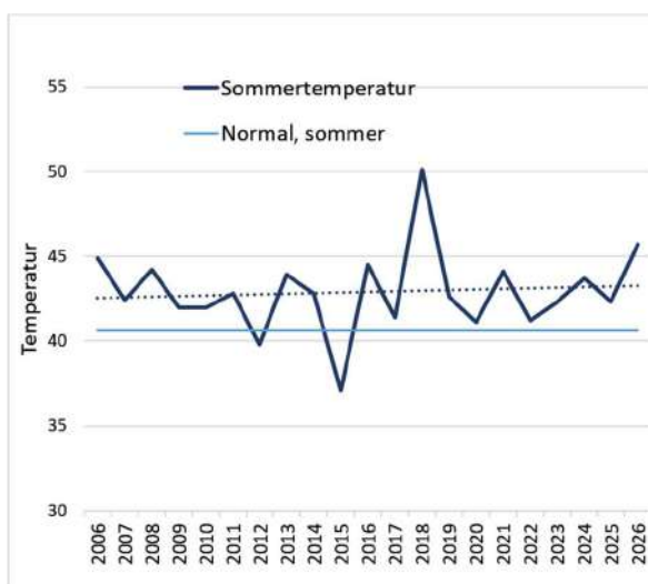
Figur 3b: Månedsmiddel temperatur (med trend) 2006-2026 og normalen summeret for månederne maj-juli.
