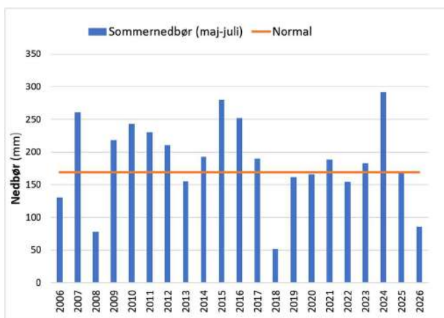
Figur 2b: Sommernedbør (summeret for maj-juli) 2006-2026 med normalen indsat.
